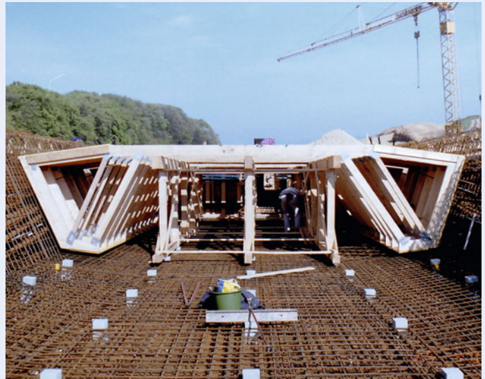
Neubau der Brücke BW 1584 im Zuge des Neubaus der Autobahn A8 Moselabstieg in Perl
